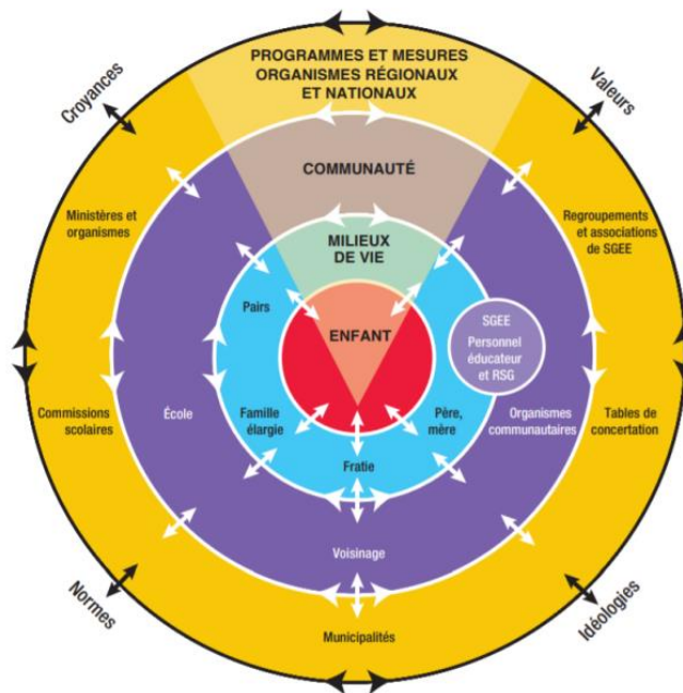
Figure 1 - L'approche écologique
