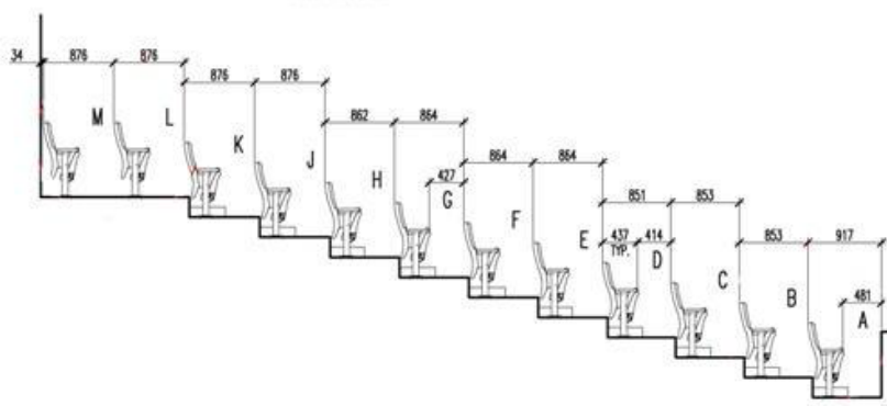
COUPE LONGITUDINALE ÉCHELLE: 1/50
