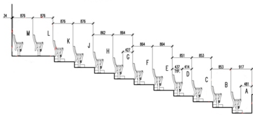
A 1 COUPE LONGITUDINALE ÉCHELLE: 1/50
